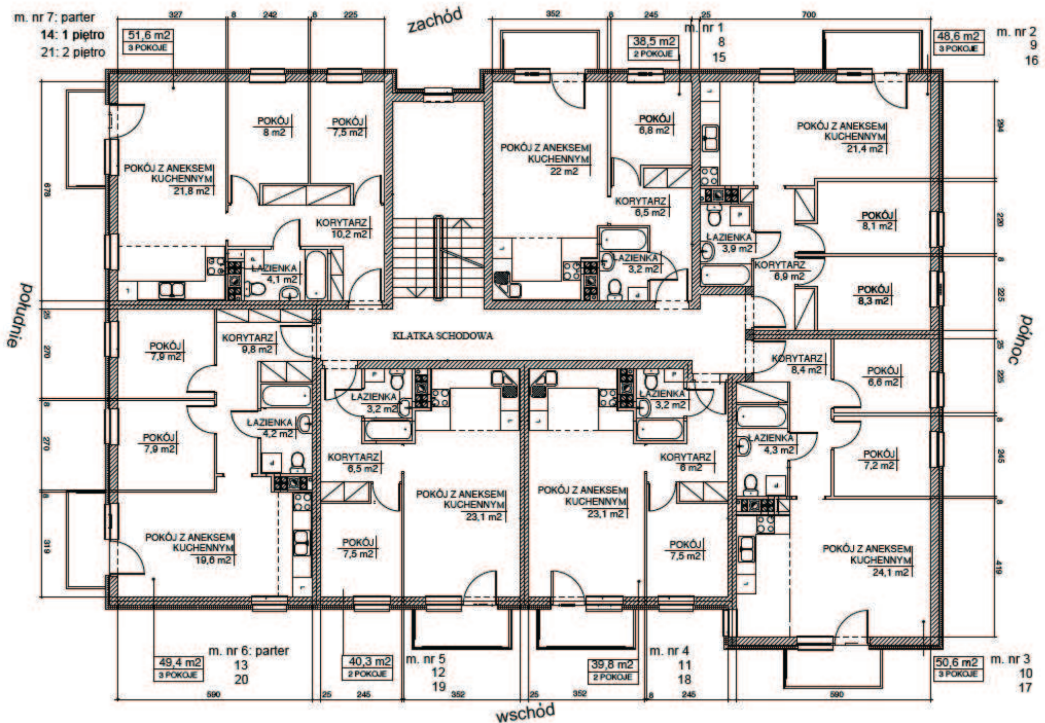
Rzut budynku nr V, ul. Dobrzyńska 4, pierwsze piętro.
